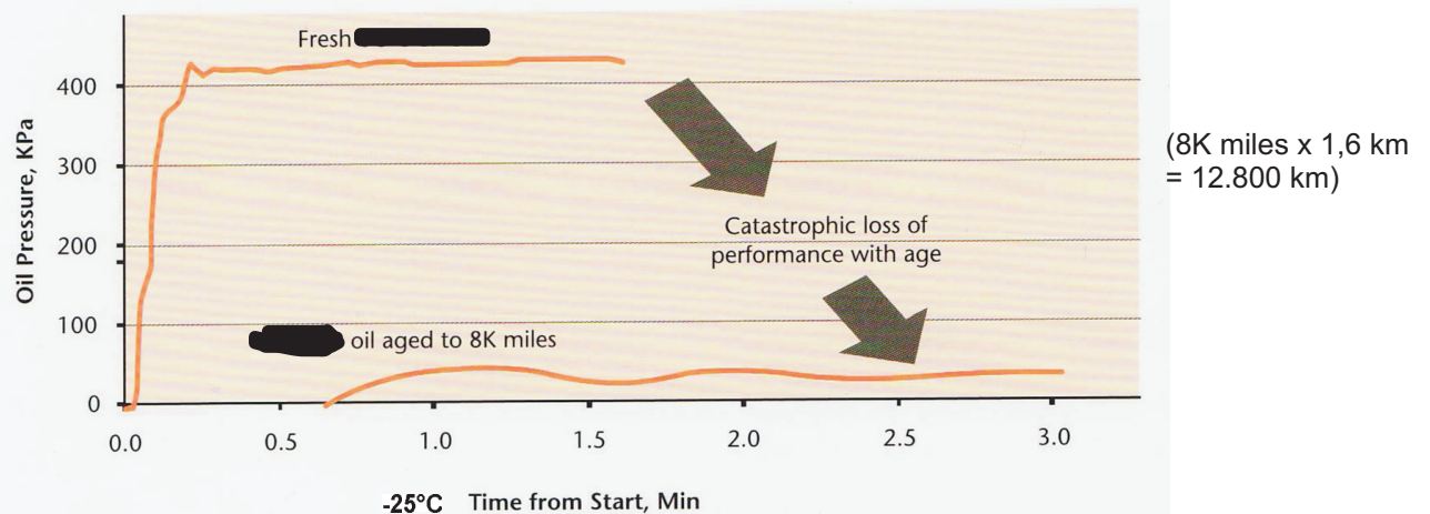
FIGURE 6 Oil Pressure Build-Up [redacted] (Huom ! tuotenimet peitetty, ettei joudu raastupaan !)
